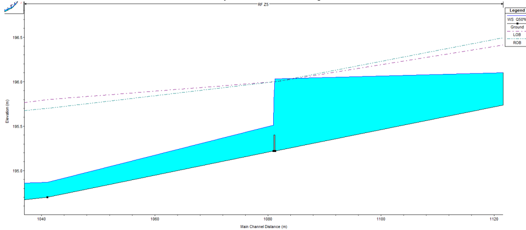
Przekrój na wlocie do zastawki Z-5:
