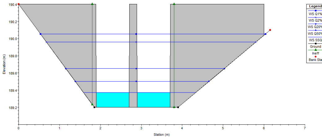
Przekrój przez przepusty zastawki PPZ-4:
