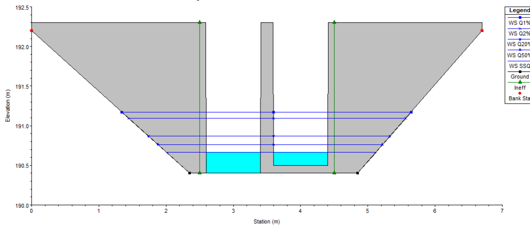
Przekrój przez przepusty zastawki PPZ-3:
