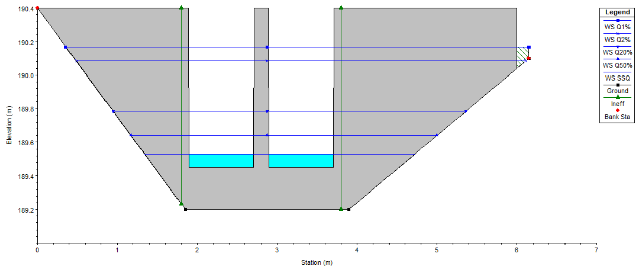
Przekrój na wlocie do zastawki PPZ-4:
