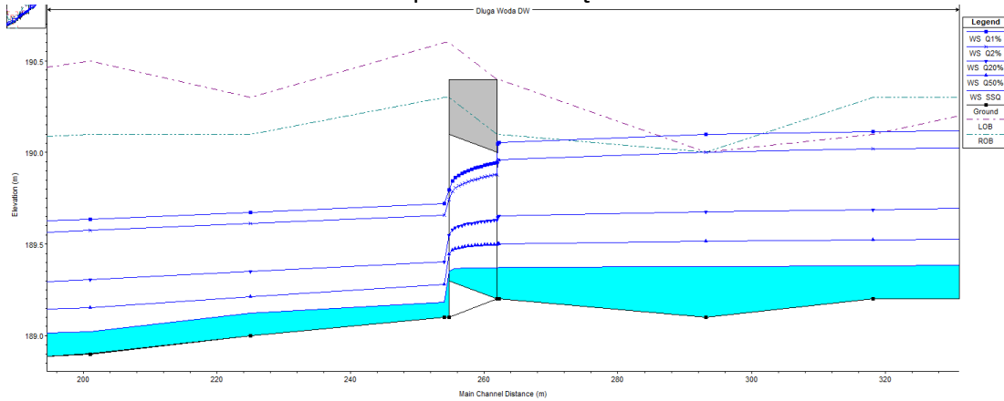
Przekrój na wlocie do zastawki PPZ-4:
