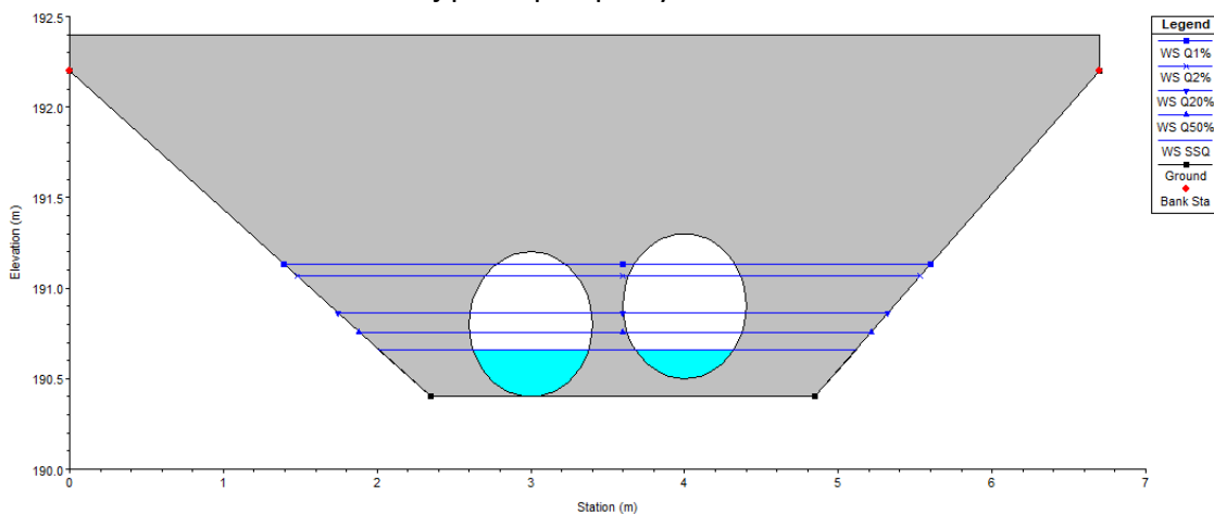
Przekrój przez przepusty zastawki PPZ-3:
