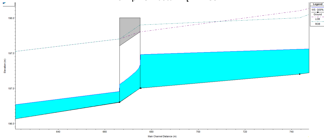
Przekrój na wlocie do zastawki PPZ-35:
