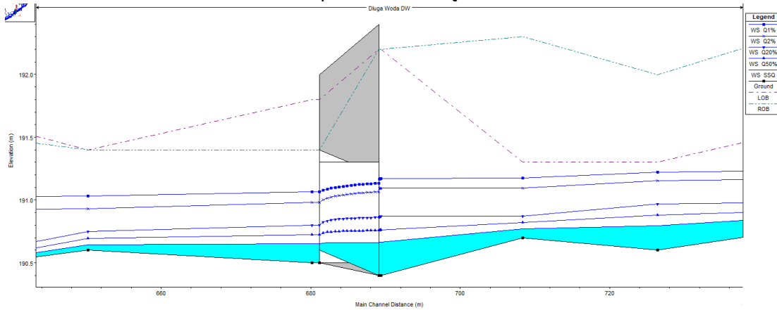
Przekrój na wlocie do zastawki PPZ-3:
